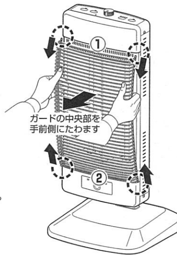
<ガードの取りはずし>
