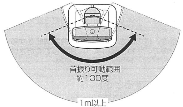
<自動首振りをするとき> (縦向きで上から見た図)
